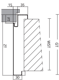
Stahlumfassungszarge Typ SUZ-M für Massivwand / Mauerwerk Bodeneinstand 40 mm
