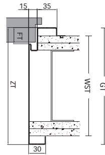
Stahlumfassungszarge Typ SUZ-L für Leichtbauwand ohne Bodeneinstand
