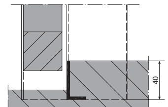
Typ FB T8510
