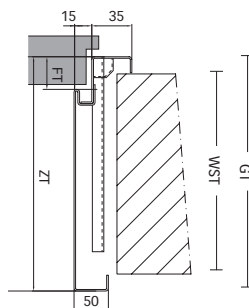
Stahlumfassungszarge Typ SUZ-Z als 2-teilige Steckzarge für Massiv- oder Leichtbauwand ohne Bodeneinstand
