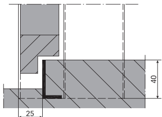
Typ S T8501
