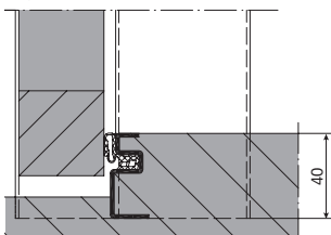
Typ DI T8502
