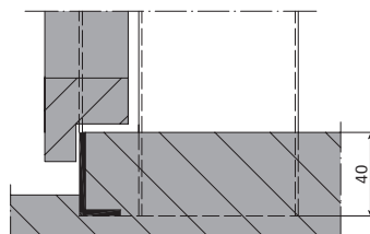
Typ SB T8509
